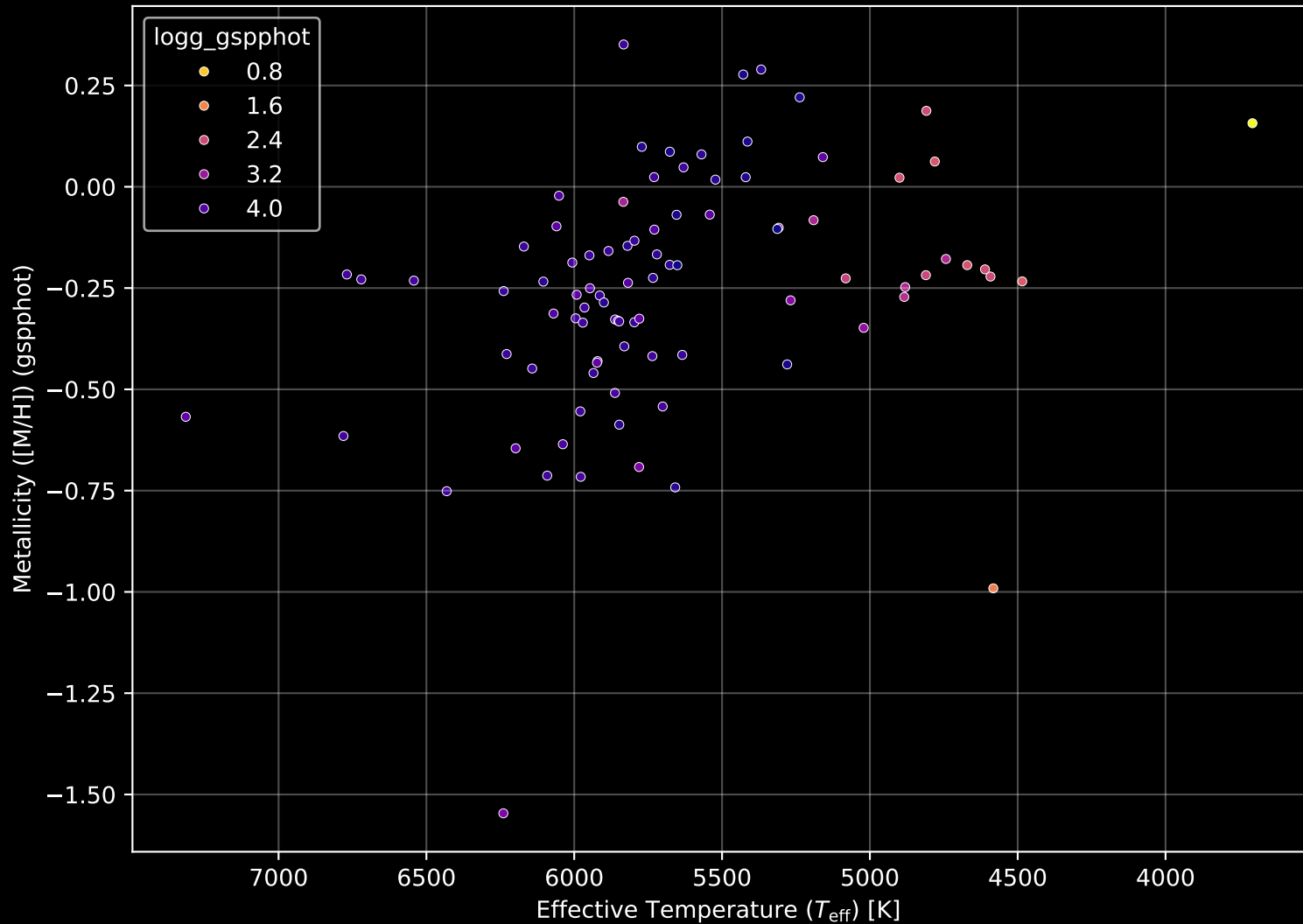
GALAH DR4 Field: [7179] Stellar Population Parameters (n= 90)
