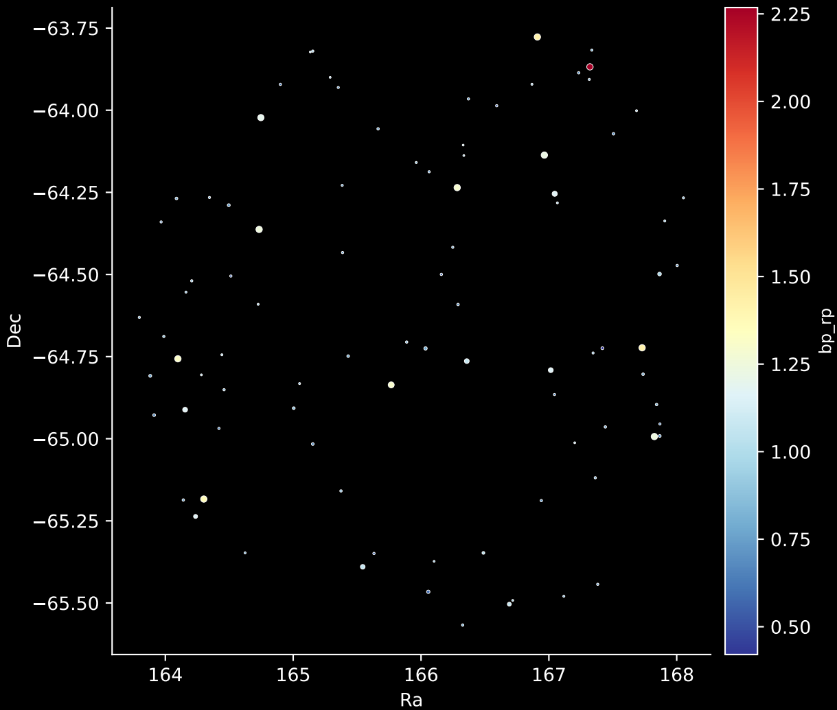
GALAH DR4 Field: [7179] Stars: 90
